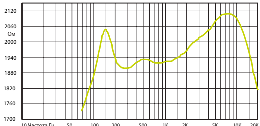
ИМПЕДАНС
