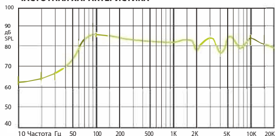
ЧАСТОТНАЯ ХАРАКТЕРИСТИКА
