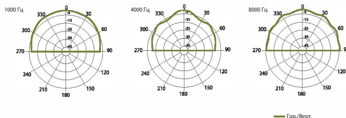
Гор./Верт. диаграммы направленности
