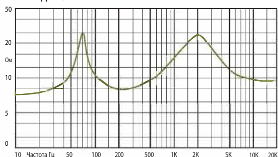
ИМПЕДАНС
