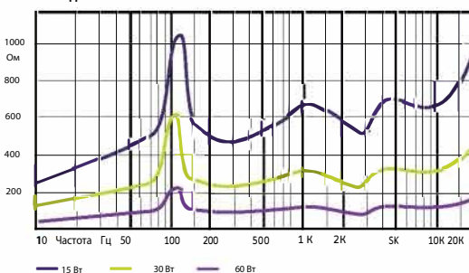
Импеданс
