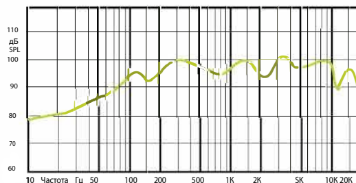
Частотная характеристика
